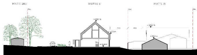
Snit DD 1:200
