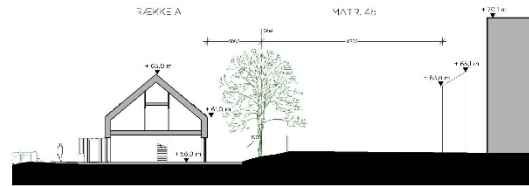
Snit AA 1:200
